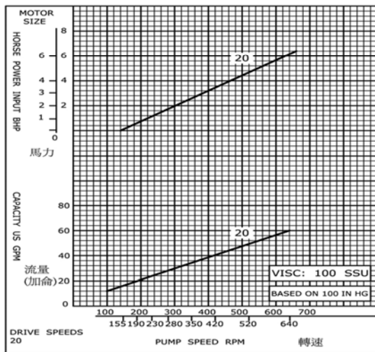
內轉齒輪泵浦輸送量參考表
